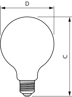
G93 230V 9-60W 806lm 2700K E27 D CL
