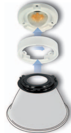
Fortimo™ SLM Modul mit CLE Dreh- und Click Ringadapter und Reflektor
